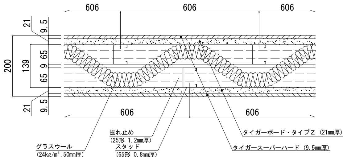
水平断面図（「A-2000・WII」遮音測定時（S-245-20参照）の壁構造）
